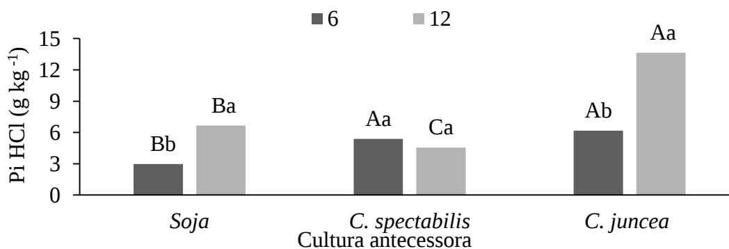
Figura 5. Interação entre culturas antecessoras (Soja, C. spectabilis e C. juncea ) à cana-de-açúcar e dose de calcário (6 e 12 Mg ha -1 ) para a variável Pi HCl (1,0 M), representante da fração não lábil, nas amostras de solo coletadas na camada de 0 a 0,1 m de profundidade na cultura da cana-de-açúcar. Caarapó – MS, 2022. Letras iguais maiúsculas indicam ausência de diferença
