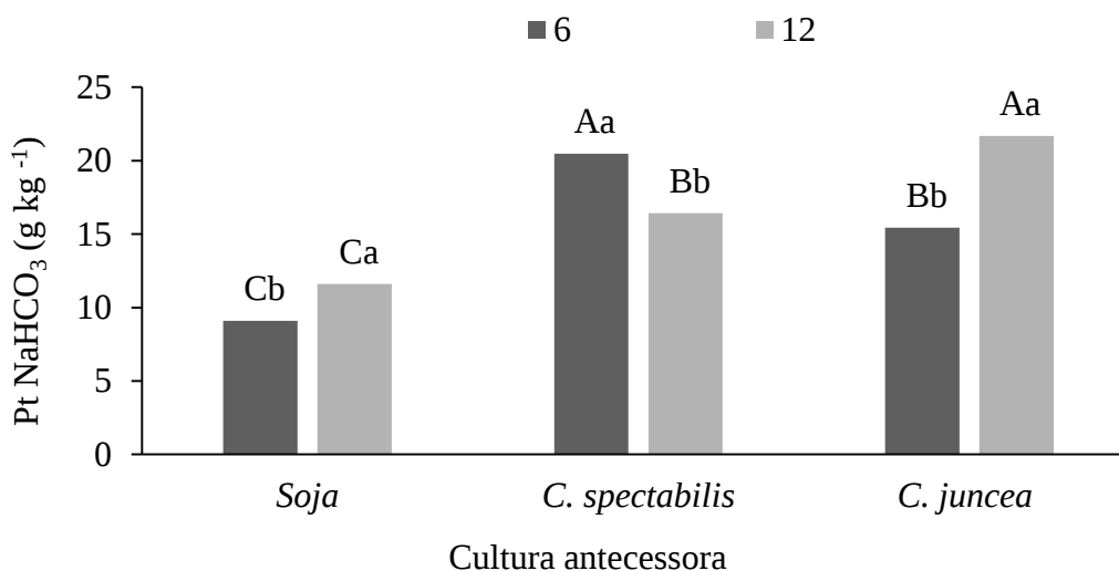
Figura 6. Interação entre (Soja, C. spectabilis e C. juncea ) à cana-de-açúcar e doses de calcário (6 e 12 Mg ha -1 ) para a variável PT NaHCO 3 (0,5 M), representante da fração lábil, nas amostras de solo coletadas na camada de 0,1 a 0,2 m de profundidade na cultura da cana-de-açúcar. Caarapó – MS, 2022. Letras iguais maiúsculas indicam ausência de diferença significativa (Tukey, 5%) para o efeito das culturas antecessoras dentro de cada dose de calcário e letras minúsculas iguais indicam ausência de diferença significativa para o efeito da dose de calcário dentro de cada cultura antecessora.
