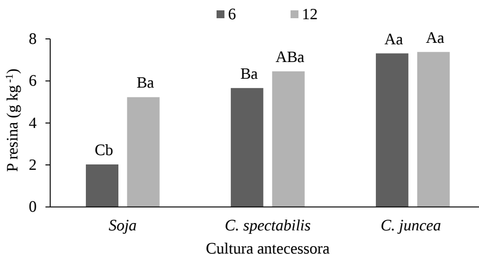
Figura 1. Interação entre cultura antecessora a cana-de-açúcar (soja, C. spectabilis e C. juncea ) e doses de calcário (6 e 12 \text{ Mg ha}^{-1} ), para a variável P resina, nas amostras de solo coletadas na camada de 0 a 0,1 m de profundidade, na cultura da cana-de-açúcar. Caarapó – MS, 2022. Letras iguais maiúsculas indicam ausência de diferença significativa (Tukey, 5%) para o efeito das culturas antecessoras dentro de cada dose de calcário e letras minúsculas iguais indicam ausência de diferença significativa para o efeito da dose de calcário dentro de cada cultura antecessora.
